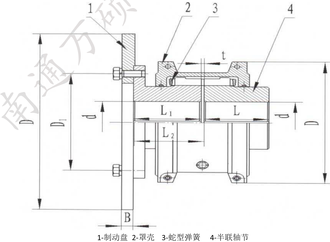
JSP 型带制动盘型蛇形弹簧联轴器（JB/T 8869-2000）
